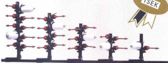
Dokuma makinaları için 2-12 iplik çıkışlı 90° veya 180° leno kerar dokuma sistemleri
