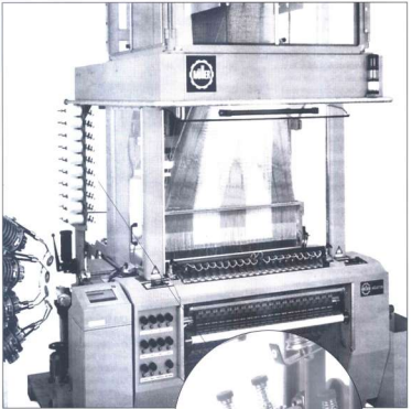
J. MÜLLER ETİKET DOKUMA MAKİNASI MUGRIP 3 VE MÜJET TİPİ İÇİN PAMUK KENAR İPLİK SİSTEMLERİ
