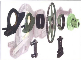
Sulzer, göçgü levent tahrik grubu komple, göçgü levent yatakları, tahrik dişileri, kare mil başlık flanşı, sıkma kelepçe flanşı, levent yataklama flanşı, orta yatak alt destek üniteleri
